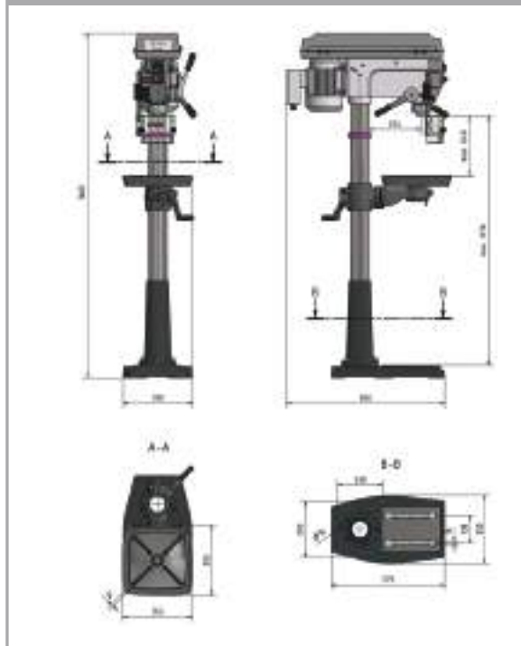
DIMENSIONI - DQ 32
